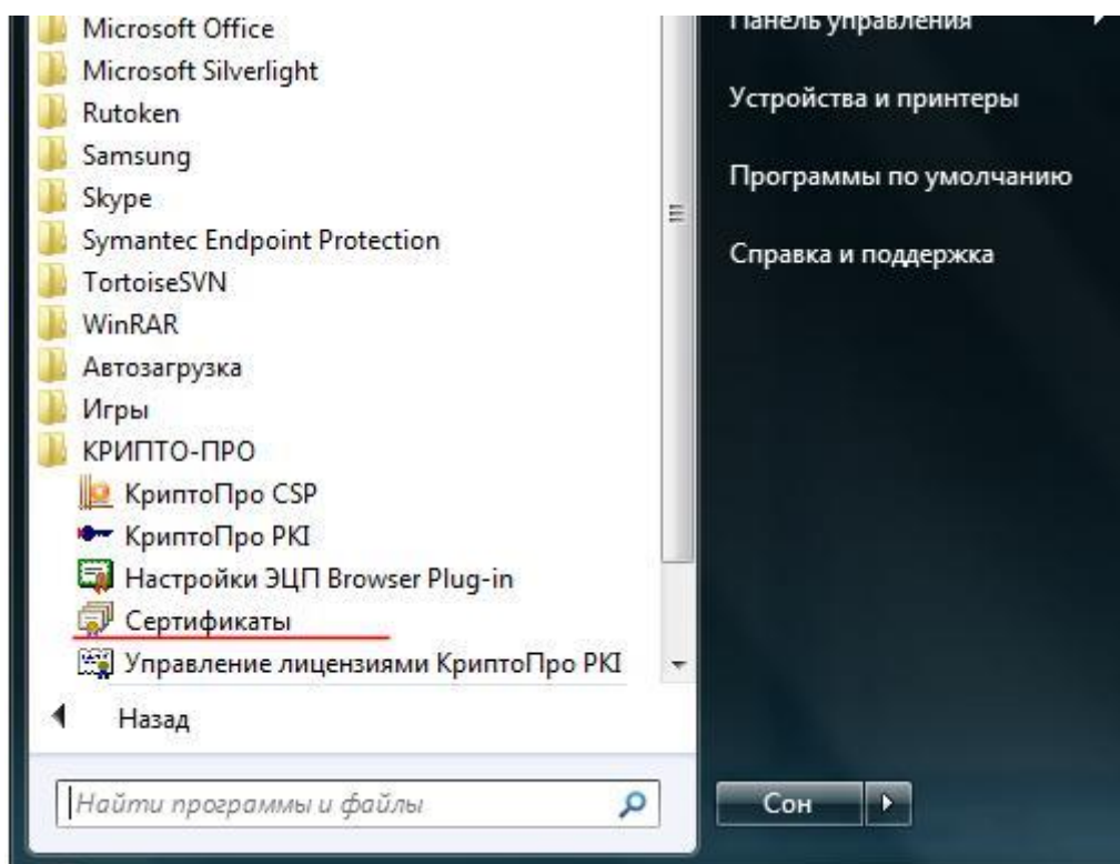
Рис. 38 – Панель «Пуск»
